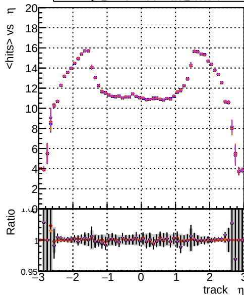
mean hits DOM CKF-test 1000evt DOM mkFitREFit-test 1000evt DOM mkFitREFit-OR-test 1000evt DOM mkFitREFit-OR4-test 1000evt
