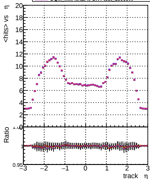
mean hits vs \eta DOM CKFit-test 1000evt DOM mkFitREFit-test 1000evt DOM mkFitREFit-OR4-test 1000evt DOM mkFitREFit-OR4-test 1000evt DOM mkFitREFit-OR4-test 1000evt
