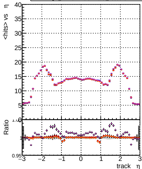
mean hits DOM CKF-test 1000evt DOM mkFitREFit-test 1000evt DOM mkFitREFit-OR4-test 1000evt DOM mkFitREFit-OR4-test 1000evt
