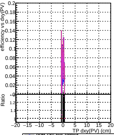
Efficiency vs Dxy(PV) DQM_CKFit-test_1000evt DQM_mkFitREFit-test_1000evt DQM_mkFitREFit-OR-test_1000evt DQM_mkFitREFit-OR-test_1000evt DQM_mkFitREFit-OR4-test_1000evt
