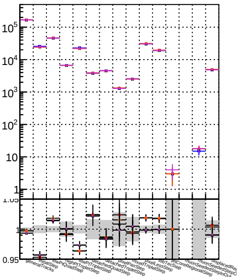
DOM CKF-test 1000evt DOM mktFitREFit-test 1000evt DOM mktFitREFit-ORK-test 1000evt DOM mktFitREFit-test 1000evt
