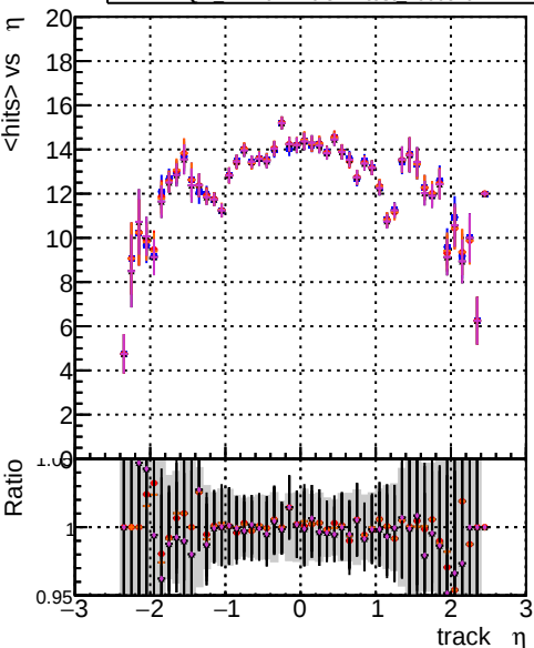
mean hits vs \eta DOM CKF-test 1000evt DOM mkFitREFit-test 1000evt DOM mkFitREFit-OR4-test 1000evt DOM mkFitREFit-OR4-test 1000evt
