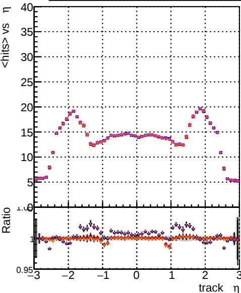
mean hits vs \eta DOM CKFit-test 1000evt DOM mkFitREFit-test 1000evt DOM mkFitREFit-OR4-test 1000evt DOM mkFitREFit-OR4-test 1000evt
