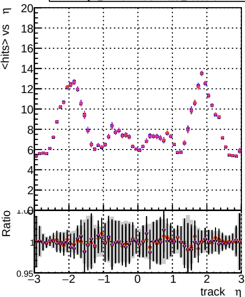
mean hits vs \eta DOM CKF-test 1000evt DOM mktFitREFit-test 1000evt DOM mktFitREFit-ORF-test 1000evt DOM mktFitREFit-ORF-test 1000evt DOM mktFitREFit-ORF-test 1000evt
