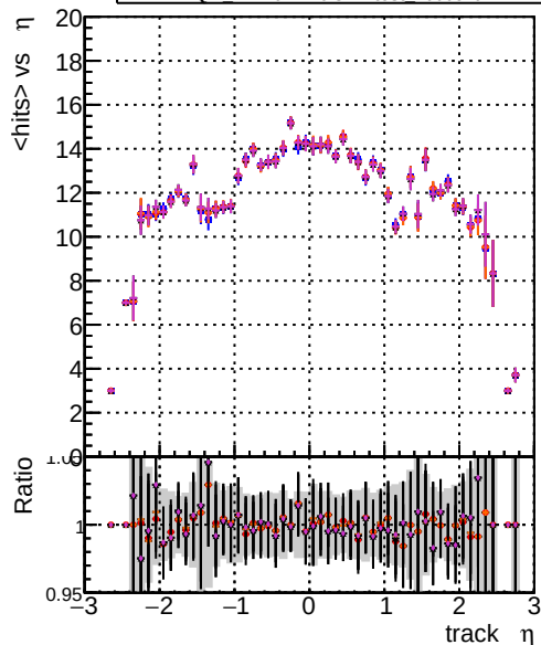
mean hits vs \eta DOM CKFit-test 1000evt DOM mkFitREFit-test 1000evt DOM mkFitREFit-OR4-test 1000evt DOM mkFitREFit-test 1000evt
