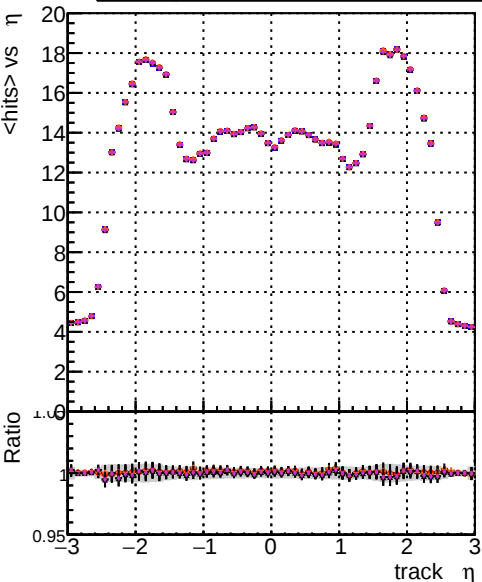
mean hits vs \eta DOM CKFit-test 1000evt DOM mkFitREFit-test 1000evt DOM mkFitREFit-OR-test 1000evt DOM mkFitREFit-ORK-test 1000evt DOM mkFitREFit-OR4-test 1000evt
