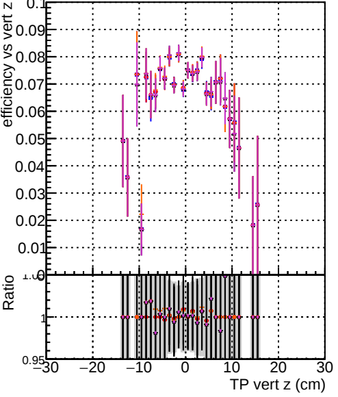
Efficiency vs vertpos DOM CKFit-testLowPt_1000evt DOM CKFit-testLowPt_10000evt DOM CKFit-testLowPt_100000evt DOM CKFit-testLowPt_1000000evt DOM CKFit-testLowPt_10000000evt DOM CKFit-testLowPt_100000000evt DOM CKFit-testLowPt_1000000000evt
