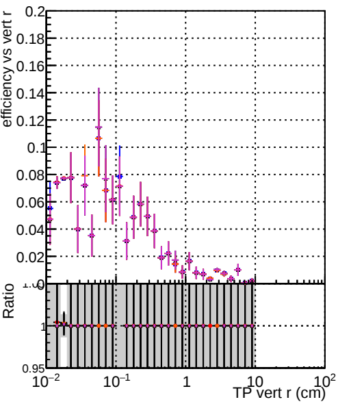
Efficiency vs vertpos DOM CKFit-testLowPt_1000evt DOM CKFit-testLowPt_10000evt DOM CKFit-testLowPt_100000evt DOM CKFit-testLowPt_1000000evt DOM CKFit-testLowPt_10000000evt DOM CKFit-testLowPt_100000000evt DOM CKFit-testLowPt_1000000000evt
