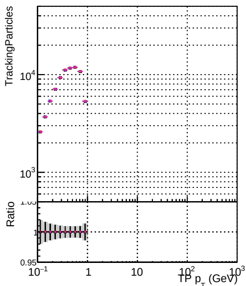
N of sim DOM CKF-testLowPt_1000evt DOM CKFREFit-testLowPt_1000evt DOM CKFREFit-OR-testLowPt_1000evt DOM CKFREFit-ORK-testLowPt_1000evt DOM CKFREFit-OR4-testLowPt_1000evt
