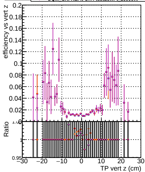
Efficiency —▲— DQM-CKFREFit-OR-testLowPt_1000evt —+— DQM-CKFREFit-ORK-testLowPt_1000evt —+— DQM-CKFREFit-OR4-testLowPt_1000evt
