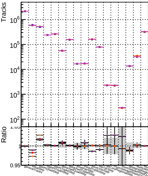
Number DOM CKF-testLowPt_1000evt DOM CKFREEfit-testLowPt_1000evt DOM CKFREEfit-OR-testLowPt_1000evt DOM CKFREEfit-ORK-testLowPt_1000evt DOM CKFREEfit-OR4-testLowPt_1000evt
