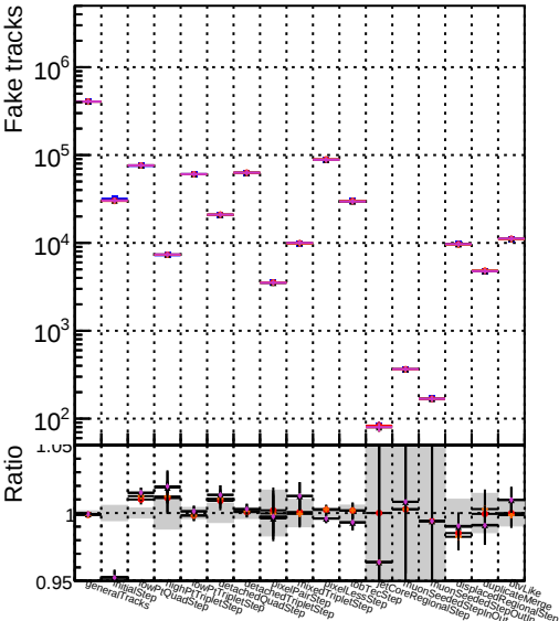
Number DOM CKF-testLowPt_1000evt DOM CKFREEfit-testLowPt_1000evt DOM CKFREEfit-OR-testLowPt_1000evt DOM CKFREEfit-ORK-testLowPt_1000evt DOM CKFREEfit-OR4-testLowPt_1000evt
