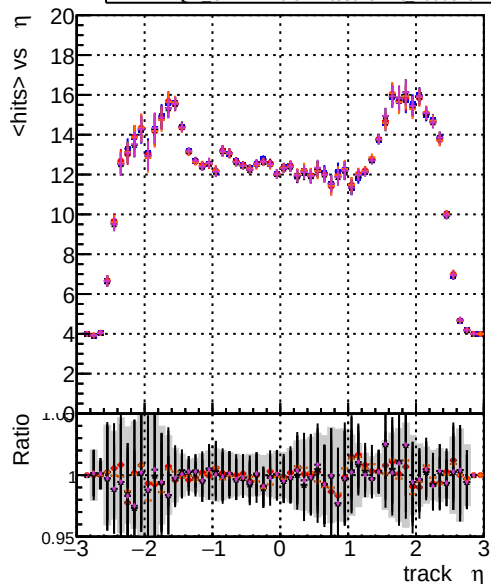
mean hits vs \eta DOM CKFit-testLowPt_1000evt DOM CKFit-testLowPt_1000evt DOM CKFit-testLowPt_1000evt DOM CKFit-testLowPt_1000evt DOM CKFit-testLowPt_1000evt
