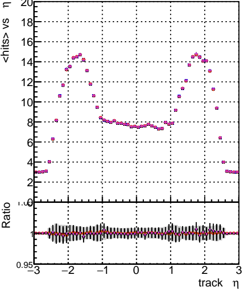
mean hits vs \eta Legend: - DQM CKFit-testLowPt_1000evt (blue) - DQM CKFit-testLowPt_1000evt (red) - DQM CKFit-testLowPt_1000evt (green) - DQM CKFit-testLowPt_1000evt (orange) - DQM CKFit-testLowPt_1000evt (purple)
