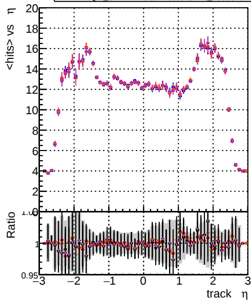
mean hits vs \eta DOM CKF-testLowPt_1000evt DOM CKF-testLowPt_1000evt DOM CKF-testLowPt_1000evt DOM CKF-testLowPt_1000evt DOM CKF-testLowPt_1000evt
