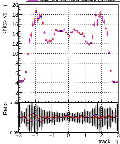
mean hits vs \eta DOM CKFit-testLowPt_1000evt DOM CKFit-testLowPt_1000evt DOM CKFit-testLowPt_1000evt DOM CKFit-testLowPt_1000evt DOM CKFit-testLowPt_1000evt DOM CKFit-testLowPt_1000evt
