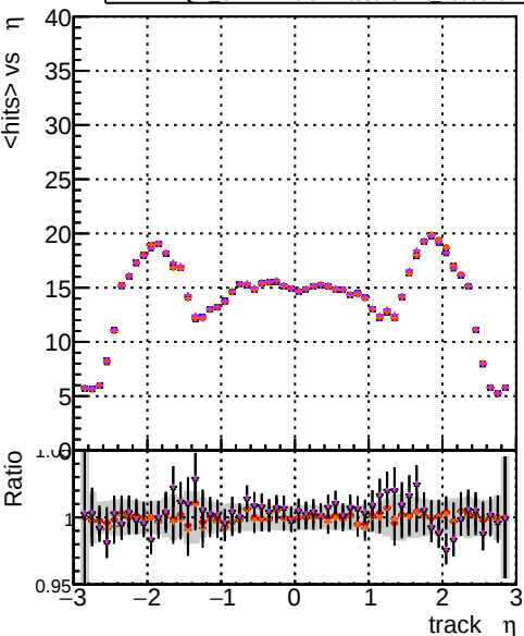
mean hits vs \eta DOM CKF-fit-LowPt_1000evt DOM CKF-fit-OR-testLowPt_1000evt DOM CKF-fit-OR4-testLowPt_1000evt DOM CKF-fit-OR4-testLowPt_1000evt
