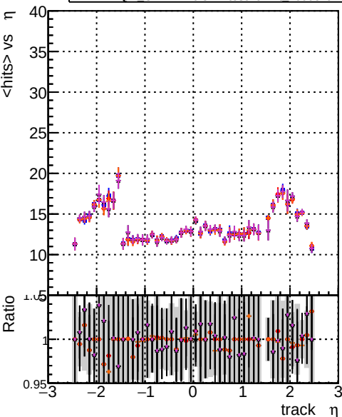
mean hits vs \eta DOM CKFit-testLowPt_1000evt DOM CKFit-testLowPt_1000evt DOM CKFit-testLowPt_1000evt DOM CKFit-testLowPt_1000evt DOM CKFit-testLowPt_1000evt
