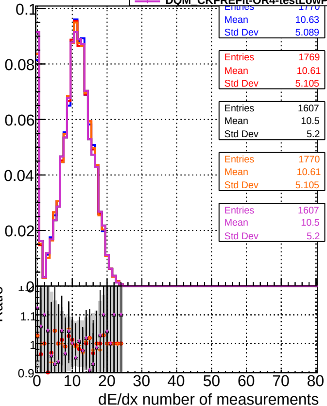
DOM CKF-testLowPt_1000evt DOM CKFREFit-testLowPt_1000evt DOM CKFREFit-OR-testLowPt_1000evt DOM CKFREFit-ORK-testLowPt_1000evt DOM CKFREFit-OR4-testLowPt_1000evt
