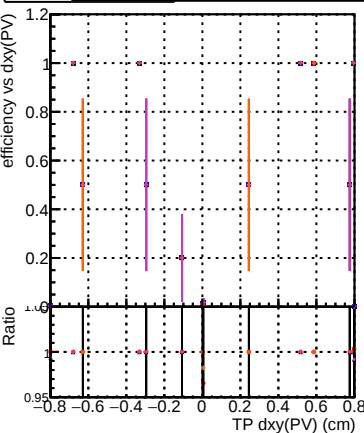
Efficiency vs Dxy(PV) Legend: DQM_CKFit-testLowPt_1000evt DQM_CKFREFit-testLowPt_1000evt DQM_CKFREFit-OR-testLowPt_1000evt DQM_CKFREFit-OR4-testLowPt_1000evt DQM_CKFREFit-OR4-testLowPt_1000evt
