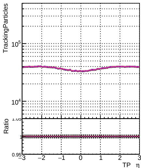
N of sin Legend Model Energy DQM-CKFREFit-OR-test LowPt 1000evt DQM-CKFREFit-ORK-test LowPt 1000evt DQM-CKFREFit-OR4-test LowPt 1000evt
