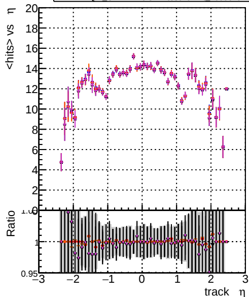
mean hits vs \eta DOM CKFit-OR4-testLowPt_1000evt DOM CKFit-OR4-testLowPt_1000evt DOM CKFit-OR4-testLowPt_1000evt DOM CKFit-OR4-testLowPt_1000evt DOM CKFit-OR4-testLowPt_1000evt
