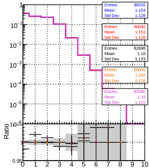
mean hits vs \eta DOM CKFit-OR4-testLowPt_1000evt DOM CKFit-OR4-testLowPt_1000evt DOM CKFit-OR4-testLowPt_1000evt DOM CKFit-OR4-testLowPt_1000evt DOM CKFit-OR4-testLowPt_1000evt
