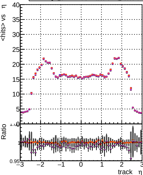
mean hits vs \eta DOM CKFit-OR4-testLowPt_1000evt DOM CKFit-OR4-testLowPt_1000evt DOM CKFit-OR4-testLowPt_1000evt DOM CKFit-OR4-testLowPt_1000evt DOM CKFit-OR4-testLowPt_1000evt
