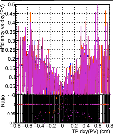
Efficiency vs Dxy(PV) DQM_CKFit-testLowPt_1000evt DQM_mkFitREFit-testLowPt_1000evt DQM_mkFitREFit-OR-testLowPt_1000evt DQM_mkFitREFit-OR2-testLowPt_1000evt
