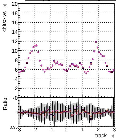
mean hits vs \eta DOM CKFit-testLowPt_1000evt DOM mkFitBEEFit-testLowPt_1000evt DOM mkFitBEEFit-OR-testLowPt_1000evt DOM mkFitBEEFit-OR2-testLowPt_1000evt DOM mkFitBEEFit-OR2-testLowPt_1000evt
