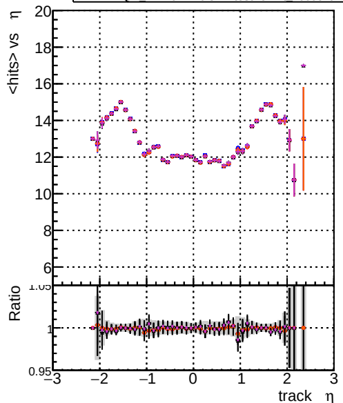
mean hits vs \eta DOM CKFit-testLowPt_1000evt DOM mkFitREFit-testLowPt_1000evt DOM mkFitREFit-OR-testLowPt_1000evt DOM mkFitREFit-OR2-testLowPt_1000evt DOM mkFitREFit-testLowPt_1000evt
