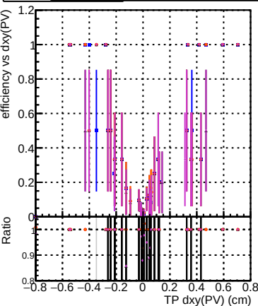
Efficiency vs Dxy(PV) Legend: DQM_CKFit-testLowPt_1000evt DQM_mkFitREFit-testLowPt_1000evt DQM_mkFitREFit-OR-testLowPt_1000evt DQM_mkFitREFit-ORK-testLowPt_1000evt DQM_mkFitREFit-OR2-testLowPt_1000evt
