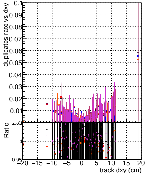
s=1000\text{eVt} s=1000\text{eVt} s=1000\text{eVt}
