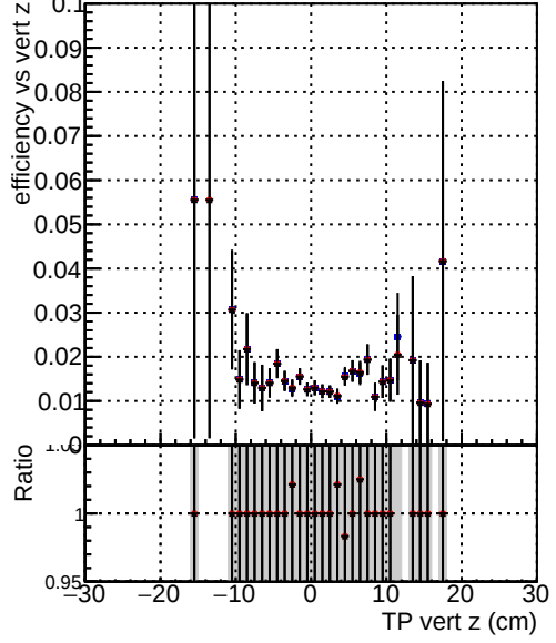
Efficiency vs. TP vert z (cm) Legend: - DQM_TT_CKF_ORIG (blue squares) - DQM_TT_CKFandPLess_ORIG (red circles) - DQM_TT_CKFandPLess_MODIF (black triangles)
