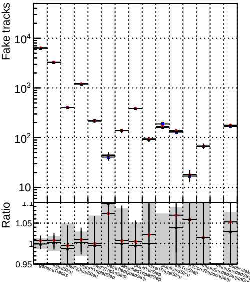
DQM_TT_CKFandPless_ORIG DQM_TT_CKFandPless_MODIF
