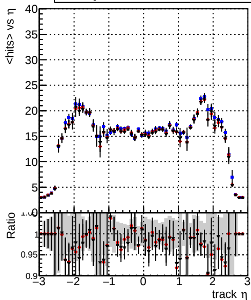
mean hits vs \eta — DQM_TT_CKF_ORIG — DQM_TT_CKFandPless_ORIG — DQM_TT_CKFandPless_MODIF
