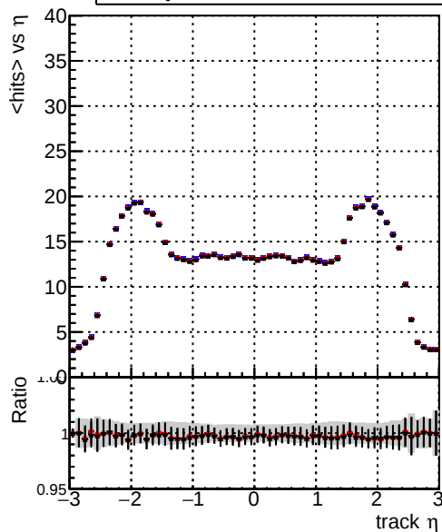
mean hit — DQM_TT_CKF_ORIG — DQM_TT_CKFandLess_ORIG — DQM_TT_CKFandLess_MODIF
