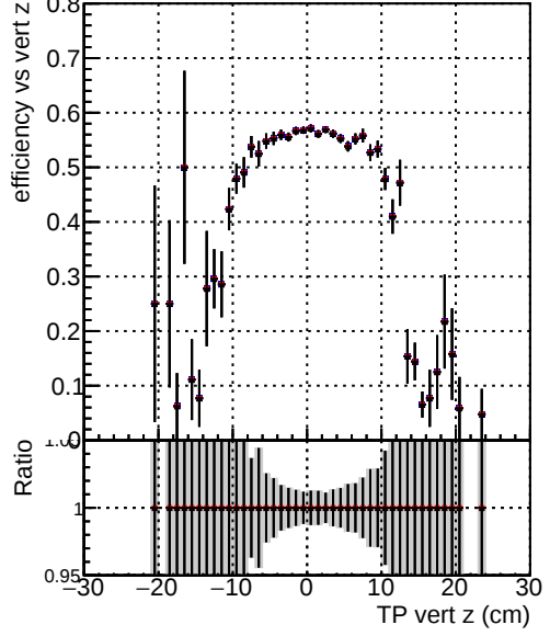
Efficiency —●— DQM_TT_CKF_ORIG —●— DQM_TT_CKFandPless_ORIG —●— DQM_TT_CKFandPless_MODIF
