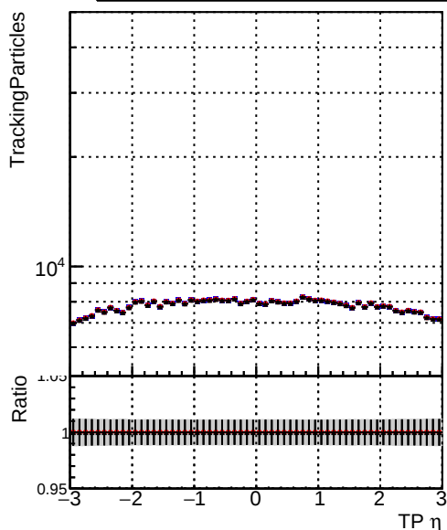
Legend: - DQM_TT_CKF_ORIG (blue dots) - DQM_TT_CKFandPLess_ORIG (red dots) - DQM_TT_CKFandPLess_MODIF (black dots)
