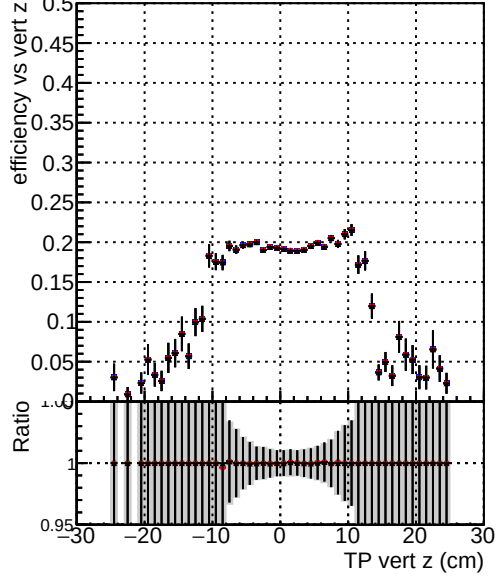
Efficiency vs. sim PV z —●— DQM_TT_CKF_ORIG —●— DQM_TT_CKFandPLess_ORIG —●— DQM_TT_CKFandPLess_MODIF
