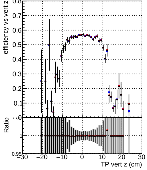
Efficiency vs. TP vert z (cm) Legend: - DQM_TT_CKF_ORIG (blue circles) - DQM_TT_CKFandPLess_ORIG (red circles) - DQM_TT_CKFandPLess_MODIF (black circles)
