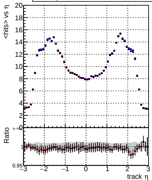
mean hits vs \eta DQM_TT_CKF_ORIG DQM_TT_CKFandPless_ORIG DQM_TT_CKFandPless_MODIF
