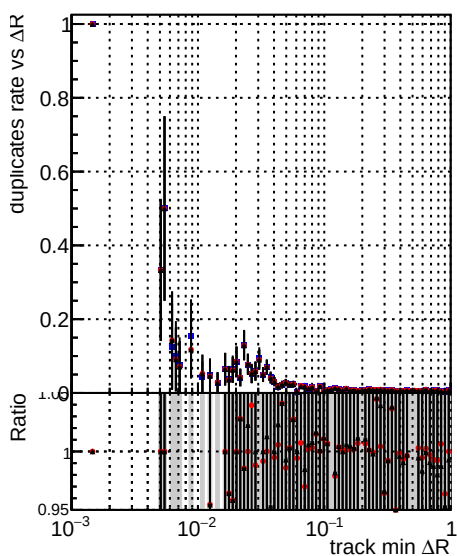
—●— DQM XiMinus original lowpt —●— DQM XiMinus newbranch lowpt pLess —●— DQM XiMinus newbranch lowpt pLessMVACand
