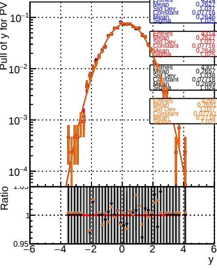
RecoPVAssoc2GenPVMatched_PullY
