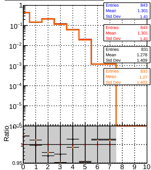
DQM_XiMinus_original_lowpt DQM_XiMinus_newbranch_lowpt DQM_XiMinus_original_lowpt_pLess DQM_XiMinus_newbranch_lowpt_pLess
