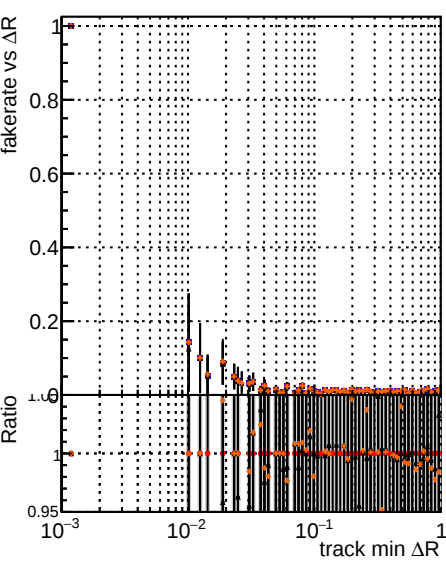
Fake rate vs \Delta R(\text{track, jet}) DQM XiMinus original lowpt DQM XiMinus newbranch lowpt DQM XiMinus original lowpt pLess DQM XiMinus newbranch lowpt pLess
