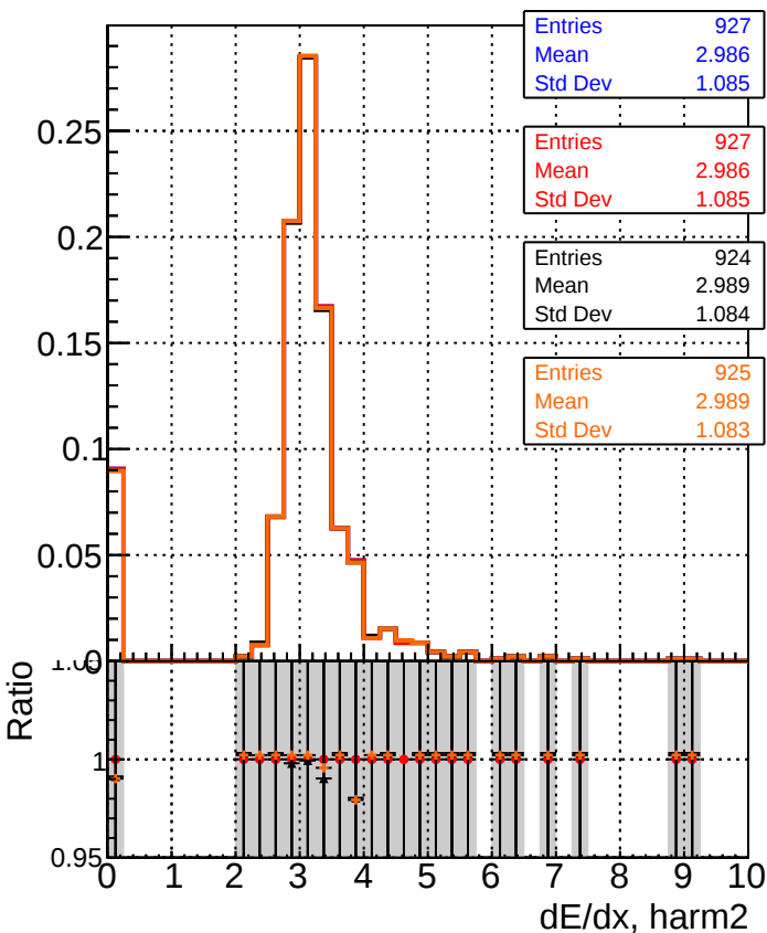
DQM_XiMinus_original_lowpt DQM_XiMinus_newbranch_lowpt DQM_XiMinus_original_lowpt_pLess DQM_XiMinus_newbranch_lowpt_pLess
