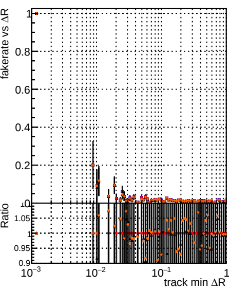
Fake rate vs \Delta R(\text{track, jet}) DQM XiMinus original DQM XiMinus newbranch DQM XiMinus original plus DQM XiMinus newbranch plus
