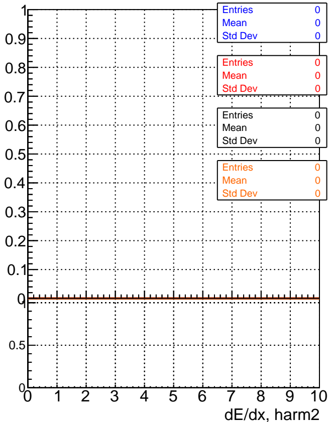
dE/dx estimator 1
