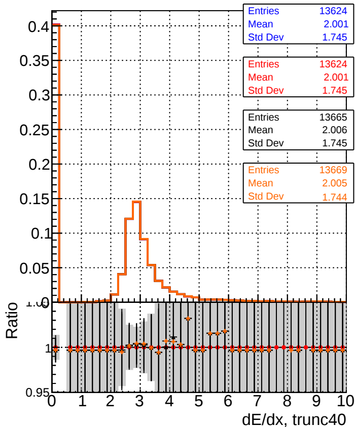
dE/dx estimator 4
