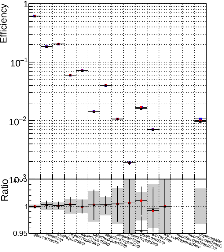
DQM TT original_lowpt DQM TT newbranch_lowpt_pLess DQM TT newbranch_lowpt_pLessMVA Cand
