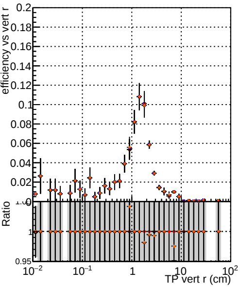
Efficiency vs vertpos — DQM TT original_lowpt — DQM TT newbranch_lowpt — DQM TT original_lowpt_pLess — DQM TT newbranch_lowpt_pLess
